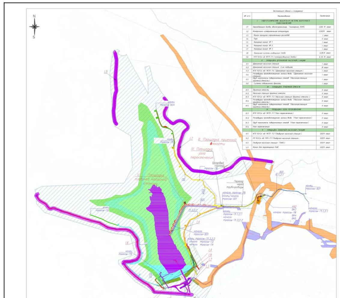
Схема расположения проектируемых зданий и сооружений в составе объекта «Золотодобывающее предприятие на месторождении «Сухой Лог». Хвостохранилище хвостов флотации»
